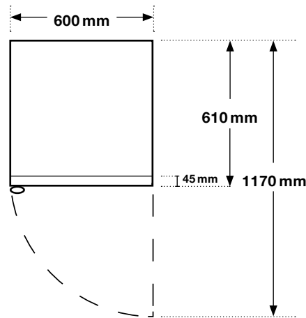
Draufsicht
